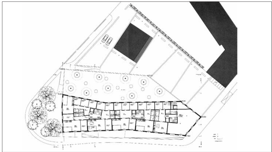
Plan du rez et des aménagements extérieurs actuels.
